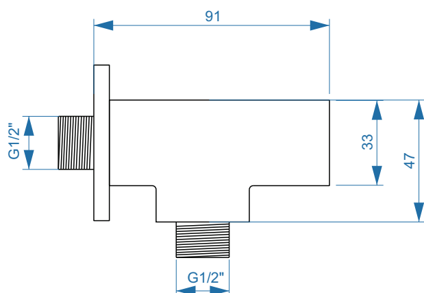
- Derivador do tubo
